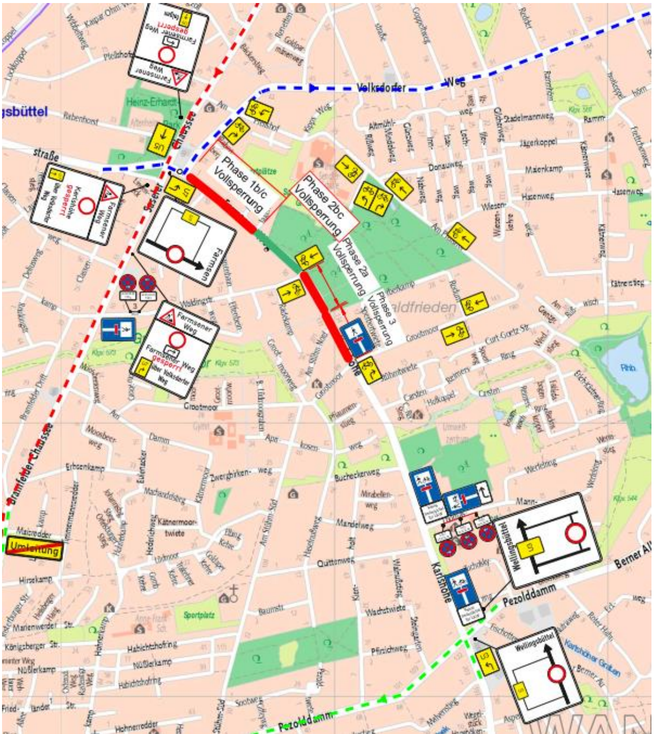
Abbildung 1: Umleitungsplan Bauabschnitt Farmesener Weg © Landesbetrieb Geoinformation und Vermessung (LGV)
