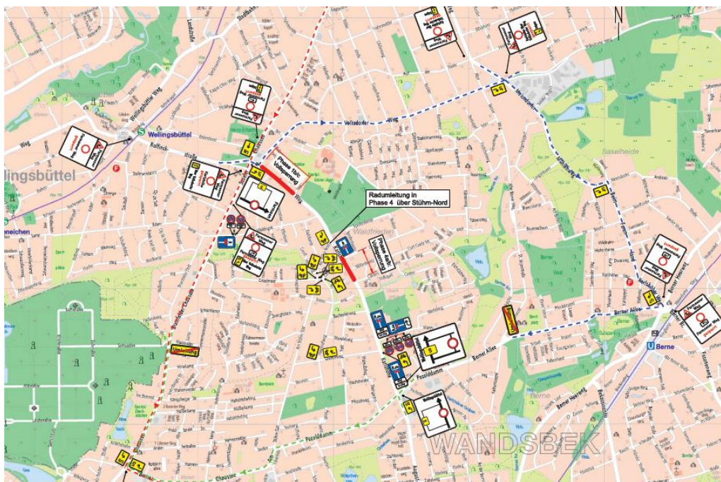
Abbildung 1: Umleitungsplan Bauabschnitt Farmsener Weg © Landesbetrieb Geoinformation und Vermessung
