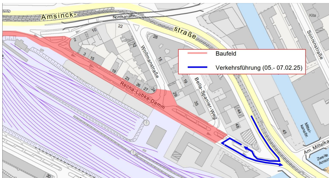
Abbildung 1: Verkehrsführung während der Sperrung der Asphaltierungsarbeiten Woltmanstraße bis Bella Spanier Weg, vom 05.02.2025 bis 07.02.2025. Quelle: www.geoportal-hamburg.de/geo-online
